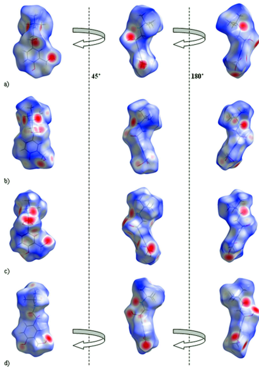
Fig. 3. Hirschfeld surfaces of: a) SB, b) SS, c) SA and d) SSU. 165x226mm (266 x 266 DPI)
